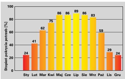
Przykładowy wykres stopnia pokrycia potrzeb energii dla podgrzewu ciepłej wody użytkowej
