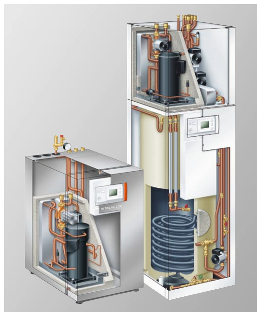
Schematyczne przekroje pompy ciepła Vitocal 200 oraz kompaktowej centrali grzewczej Vitocal 343.
