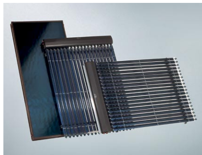
Kolektory firmy Viessmann od kilkunastu lat spełniają rygorystyczne wymagania jakościowe, obecnie zawarte w normie europejskiej i zarazem polskiej PN-EN 12975.
